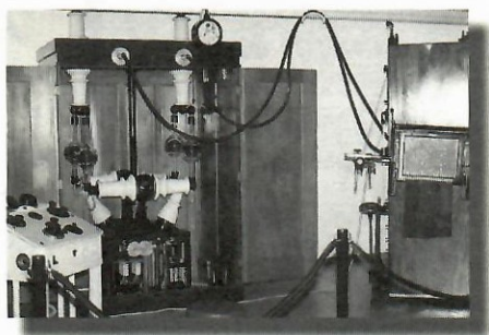
APARELL CLÀSSIC DE RAIG X QUE FOU DEL METGE AGUSTÍ PEDRO I PONS (UB CAMPUS DE BELLVITGE)
